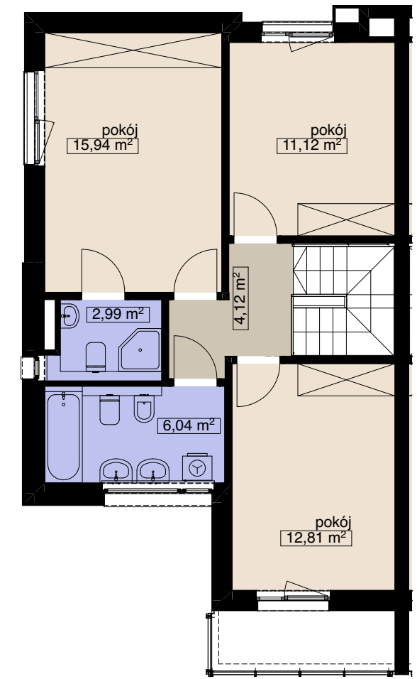
RZUT 1. PIĘTRA
