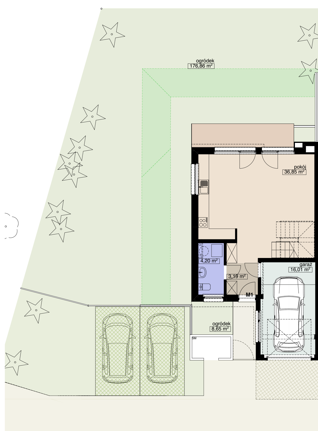
RZUT PARTERU
